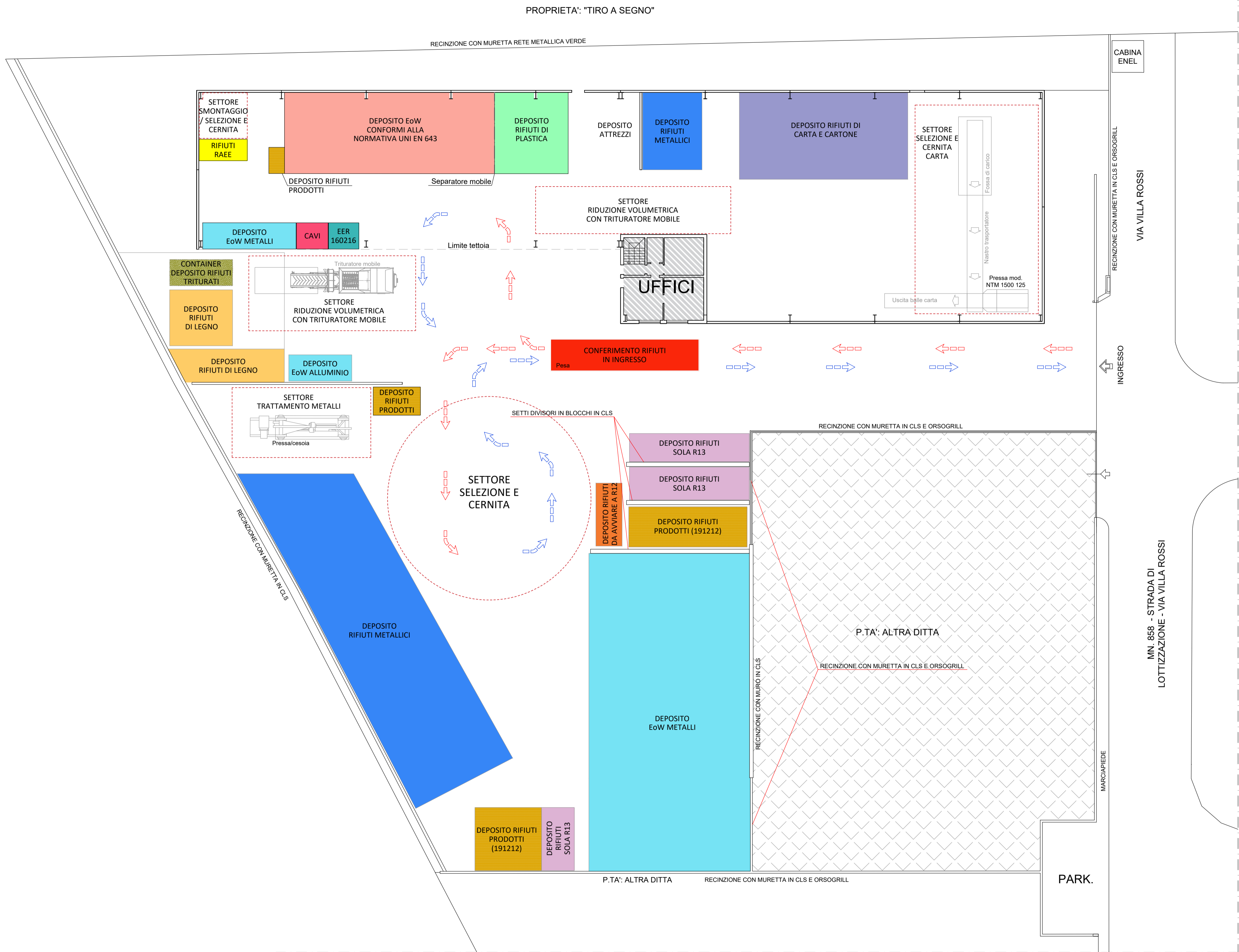
PLANIMETRIA GENERALE LAYOUT ORGANIZZATIVO IMPIANTO SCALA 1:200
