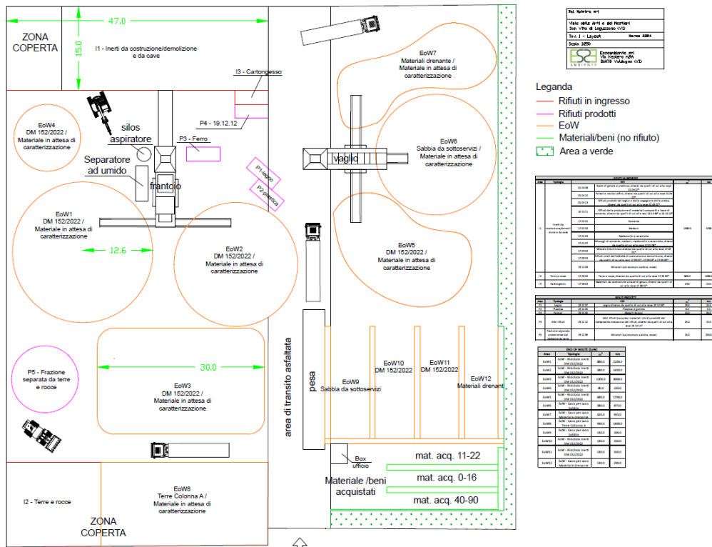
Planimetria generale di impianto (Allegato grafico 1 Layout)
