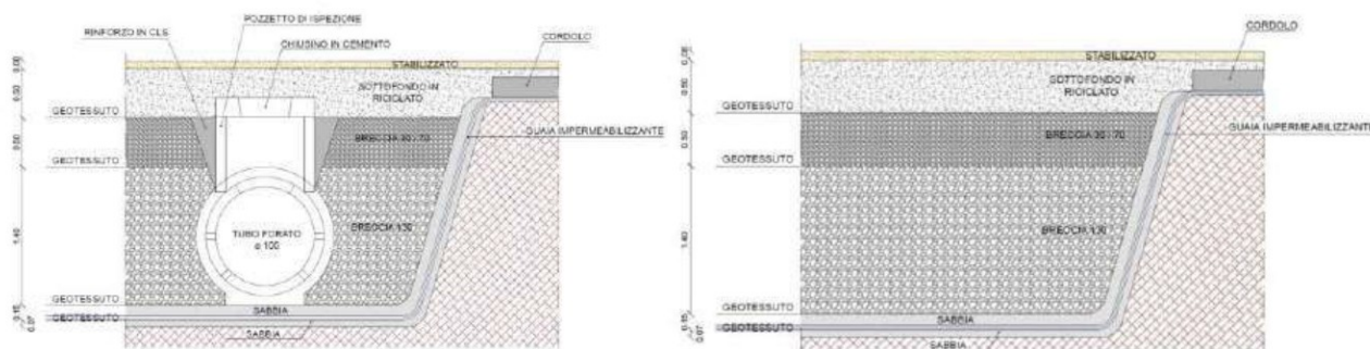
Tipologie previste delle stratigrafie atte a realizzare il volume di laminazione
