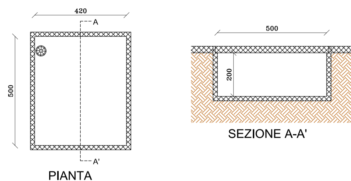
PARTICOLARE VASCA 6 SCALA 1:100
