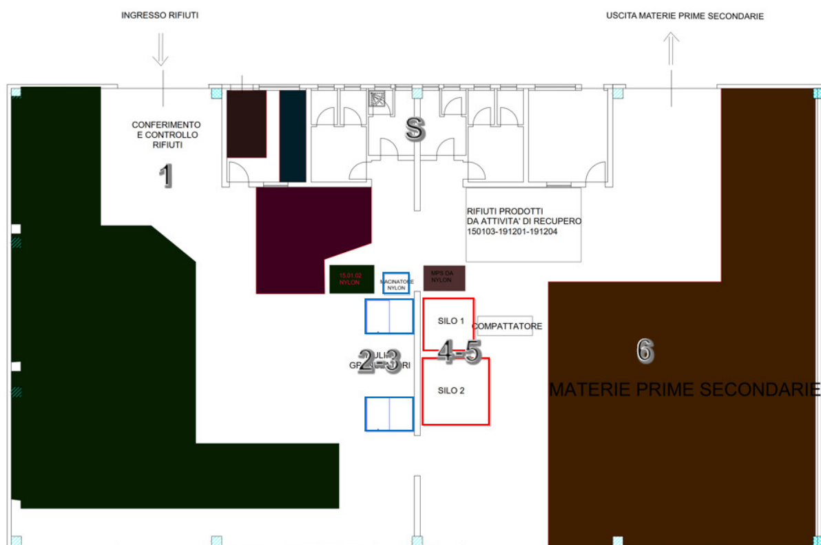
Figura 3-1. Estratto tavola "Layout rifiuti"
