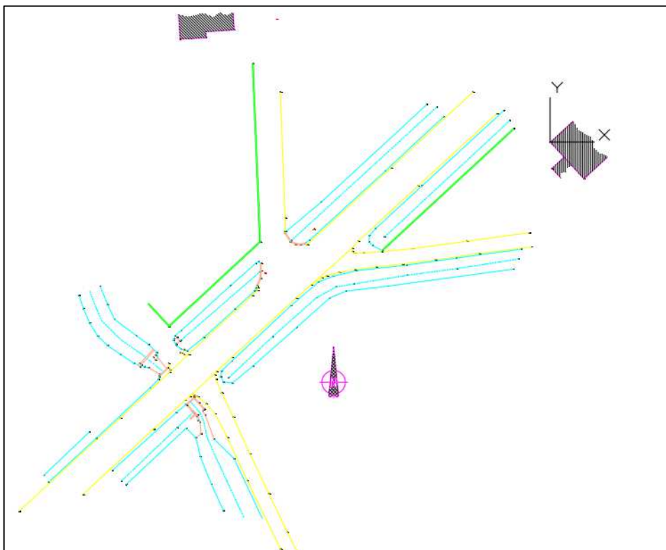
Rilievo dell'intersezione est (sopra) ed ovest (sotto) di Via Piazzola (laterali) sulla S.P. n. 24
