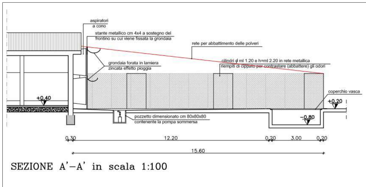
Particolare del sistema per l'abbattimento degli odori e delle polveri
