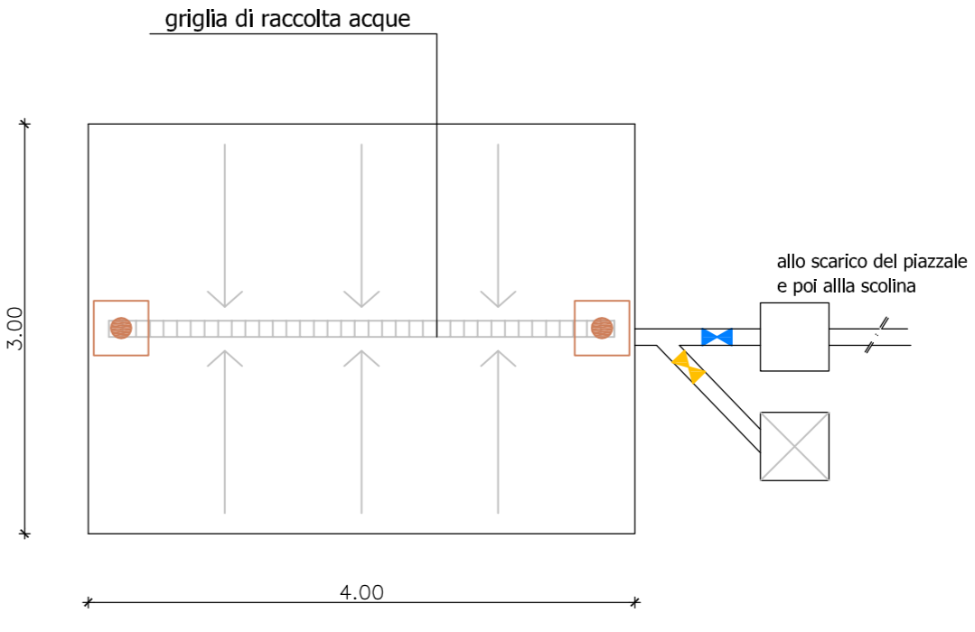
PARTICOLARE PIAZZOLA DI DISINFESTAZIONE in scala 1:50
