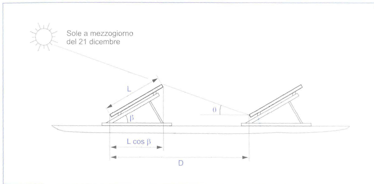
Distanza D tra schiere di moduli tale da evitare l'ombra a mezzogiorno del 21 dicembre (solstizio invernale)
