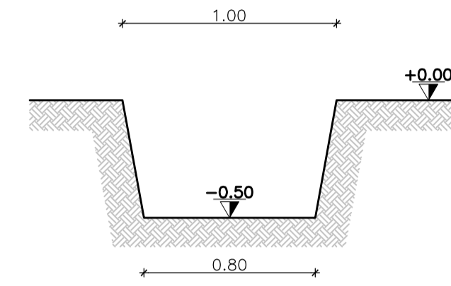
SEZIONE D-D DELLA SCOLINA in scala 1:25
