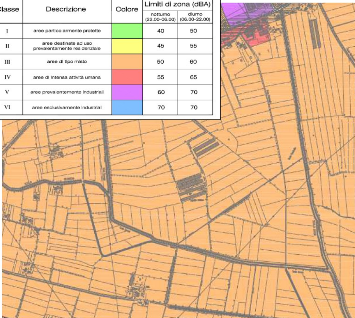
- estratto zonizzazione acustica comune di Villaga (VI) -
