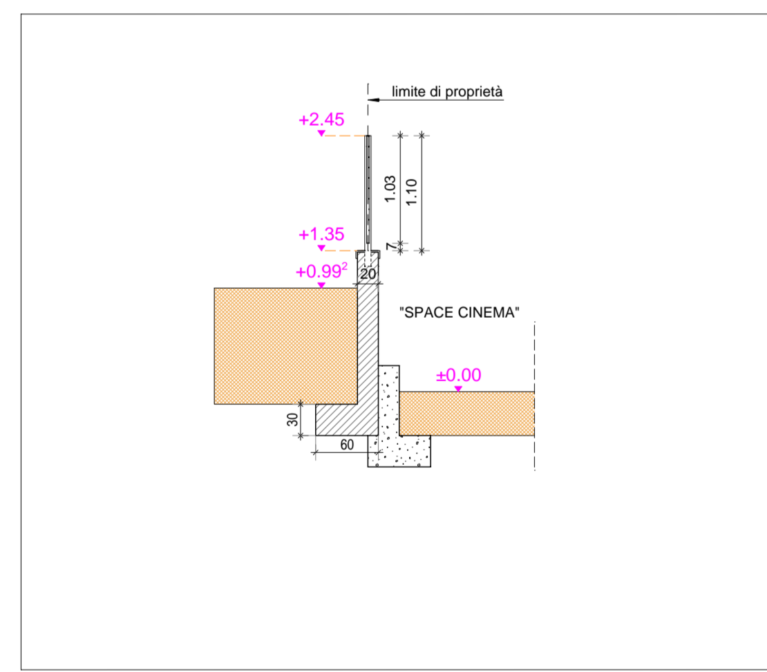
SEZ. A-A RIFERITA ALLA RECINIZIONE SITUATA AL CONFINE CON "SPACE CINEMA" SCALA 1:50
