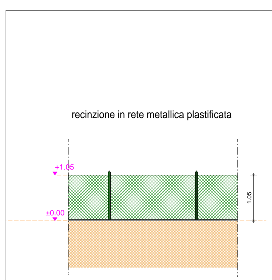
PARTICOLARE DI RECINIZIONE SITUATA AL CONFINE CON L'AUTOSTRADA SCALA 1:50
