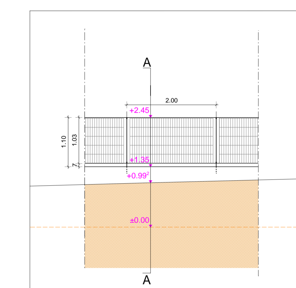
PARTICOLARE DI RECINIZIONE SITUATA AL CONFINE CON "SPACE CINEMA" SCALA 1:50
