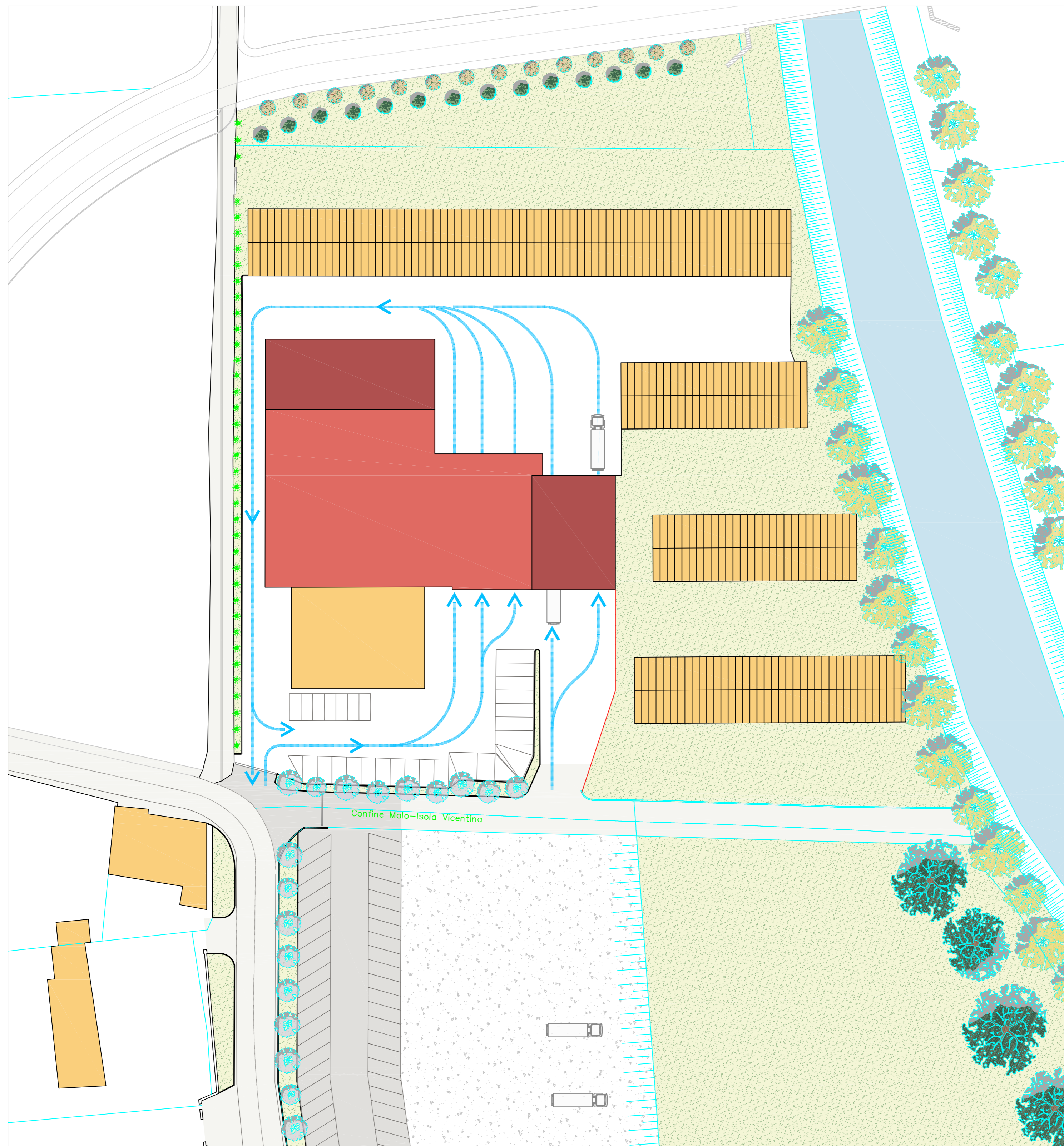
PLANIMETRIA SCALA 1:500 - INQUADRAMENTO TERRITORIALE E VIABILITA' INTERNA
