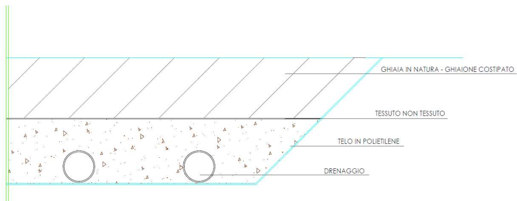
Figura 2. Particolare del fondo dell'invaso.
