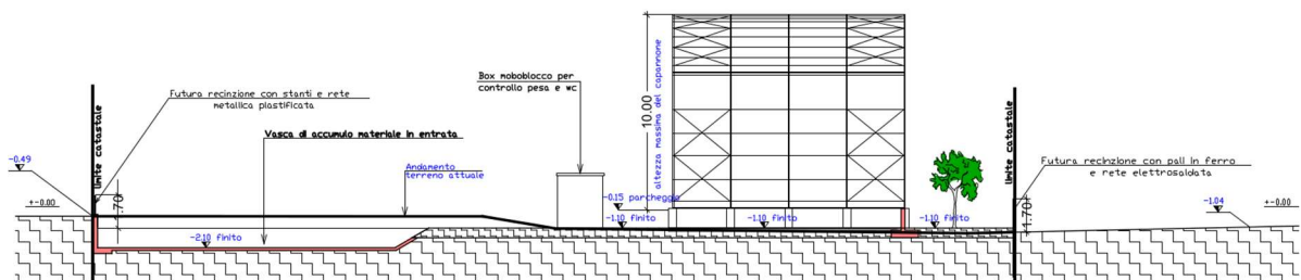
Figura 1. Sezione dell'area dell'impianto.
