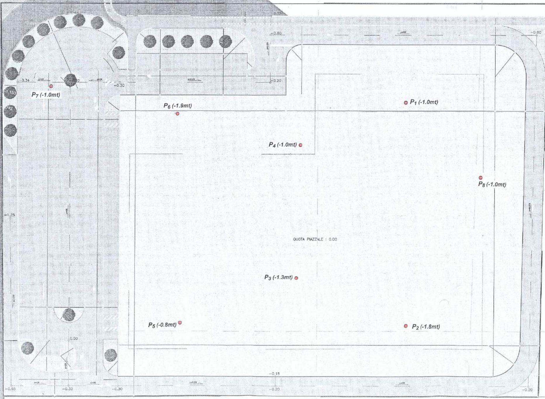
TAV.3 – Ubicazione delle Prove Penetrometriche su planimetria di progetto alla scala 1:500 con indicazione delle profondità del substrato ghiaioso dal p.c. attuale
