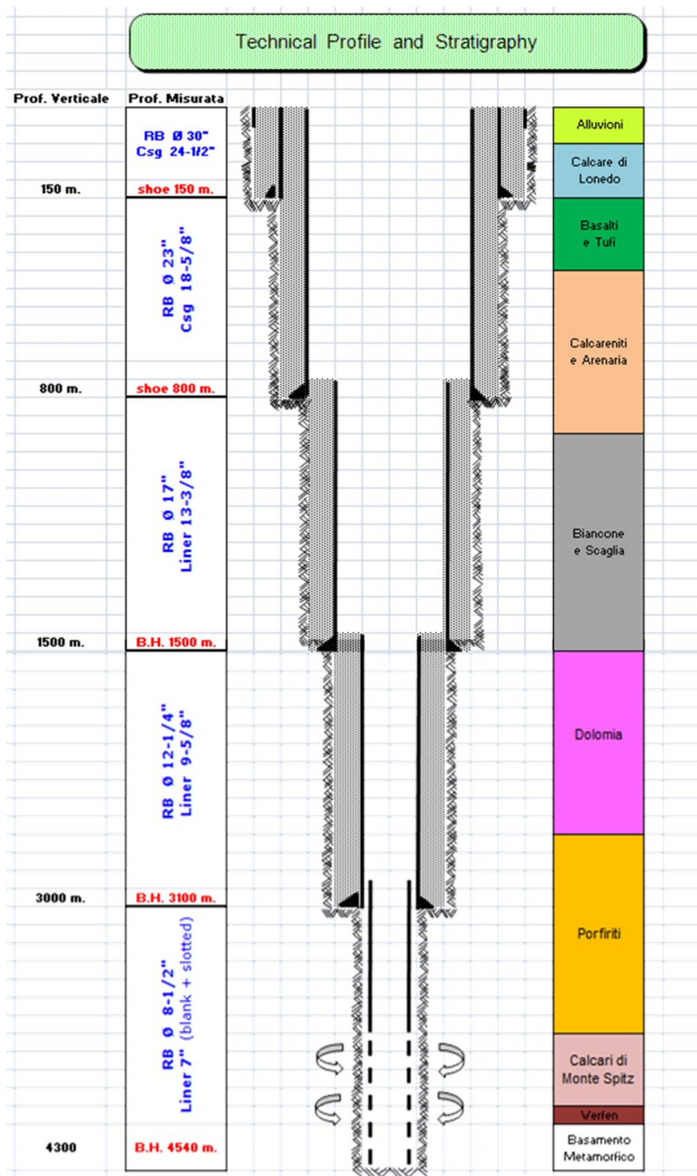
Fig. 11 -- Previsione stratigrafica e rivestimento ipotizzato dei sondaggi oggetto del presente progetto
