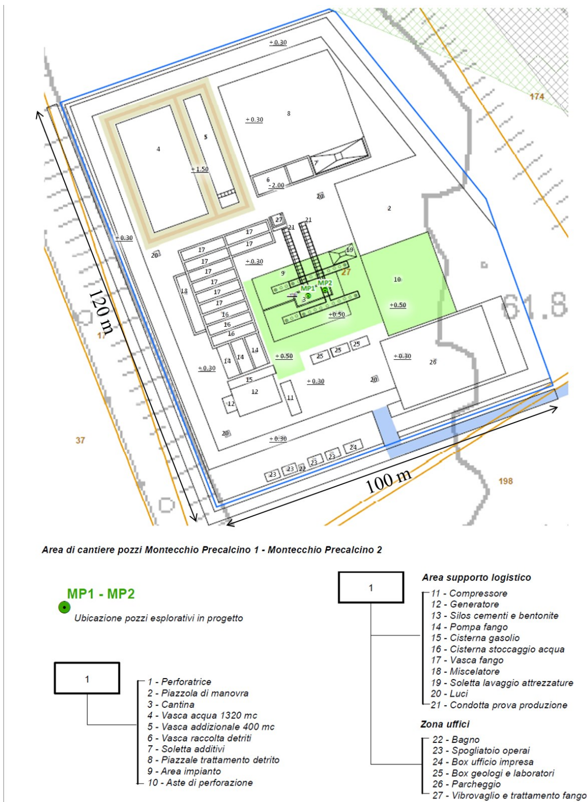
Fig. 8 - Localizzazione planimetrica di insieme delle opere previste
