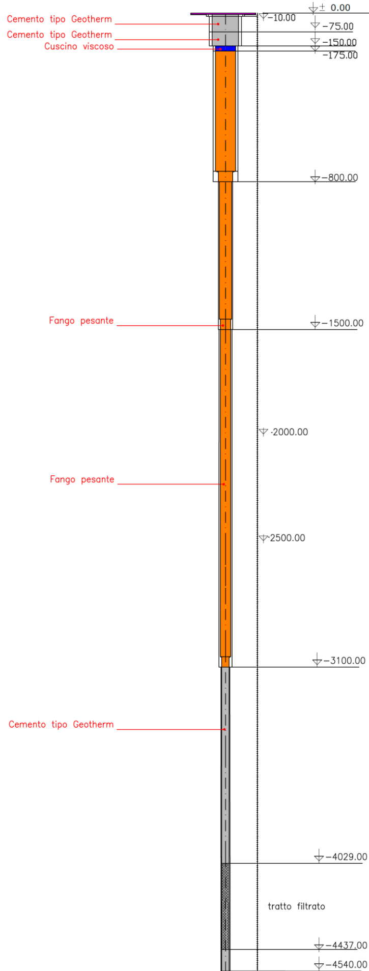
Fig. 12. Schema di chiusura mineraria del pozzo
