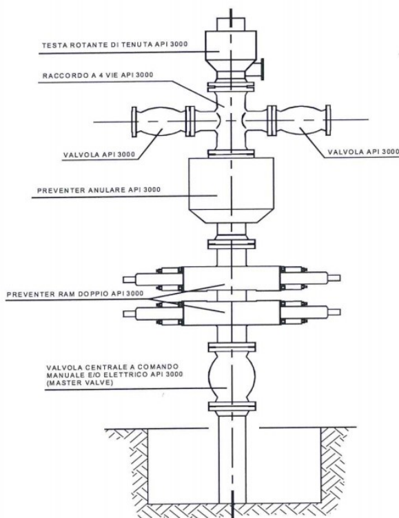
Fig. 10 - Configurazione di testa pozzo in fase di perforazione
