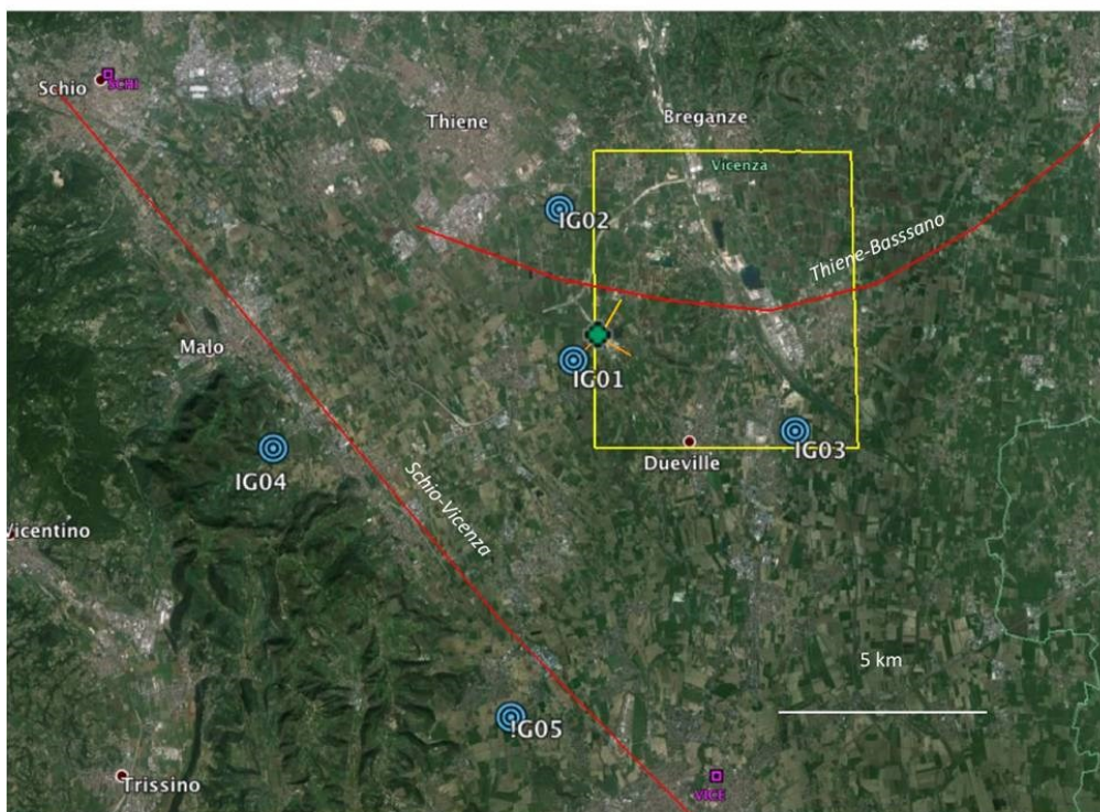
Fig. 27 - Disposizione delle stazioni prevista per la Rete Sismica di Montecchio, a scala locale. I simboli rappresentano: quelli rotondi azzurri le stazioni della rete proposta (sigla IG), il rombo verde la posizione dei pozzi con le due deviazioni orizzontali in profondità (segmenti arancio), il rettangolo giallo i limiti della concessione, la linea bianca in basso la distanza di 5 km. I simboli piccoli colore magenta, rappresentano le posizioni delle stazioni GPS permanenti del Veneto già presenti nell'area.
