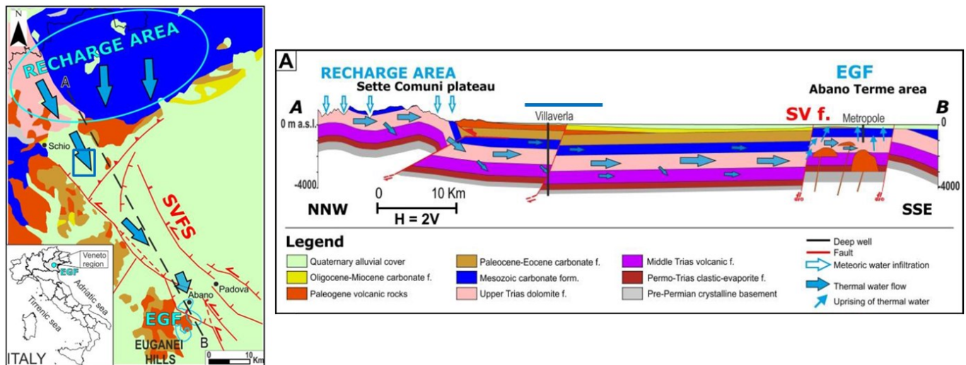
Fig. 20 - Modello concettuale e sezione NW-SE estratta e modificata con l'ingombro del P.R. da Pola et al., (2013).
