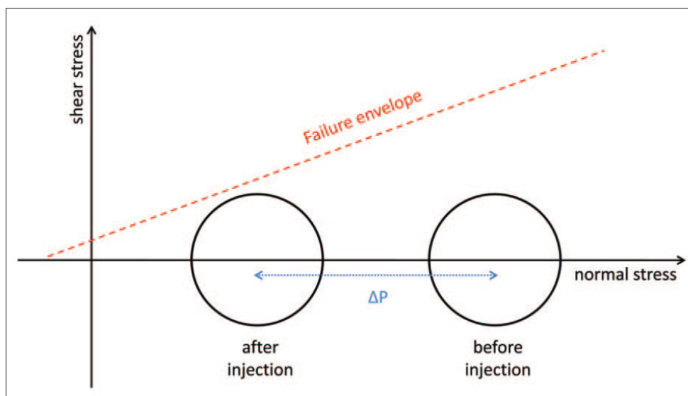
Fig. 29 . Diagramma di Mohr-Coulomb che illustra come l'iniezione di fluidi diminuisca il campo di stress (estratto da Suckale, 2010)
