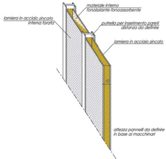
PARTICOLARE PARETE A SANDWICH FONOIOLANTE-FONOASSORBENTE SCALA 1:20 pannelli da m.2.00 per 10 cm. di spessore
