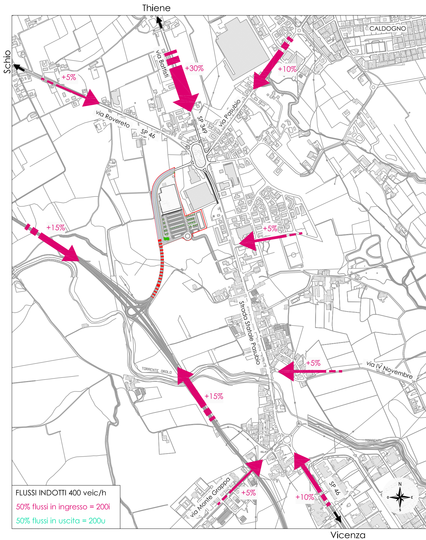
INTERSEZIONE 1 - FLUSSI INDOTTI
