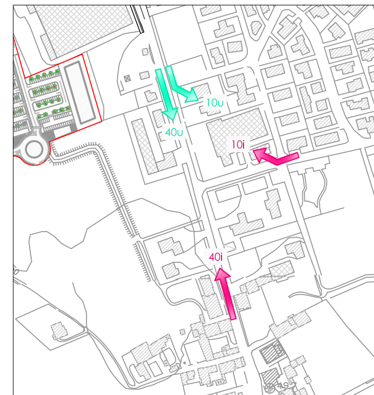
INTERSEZIONE 4 - FLUSSI INDOTTI
