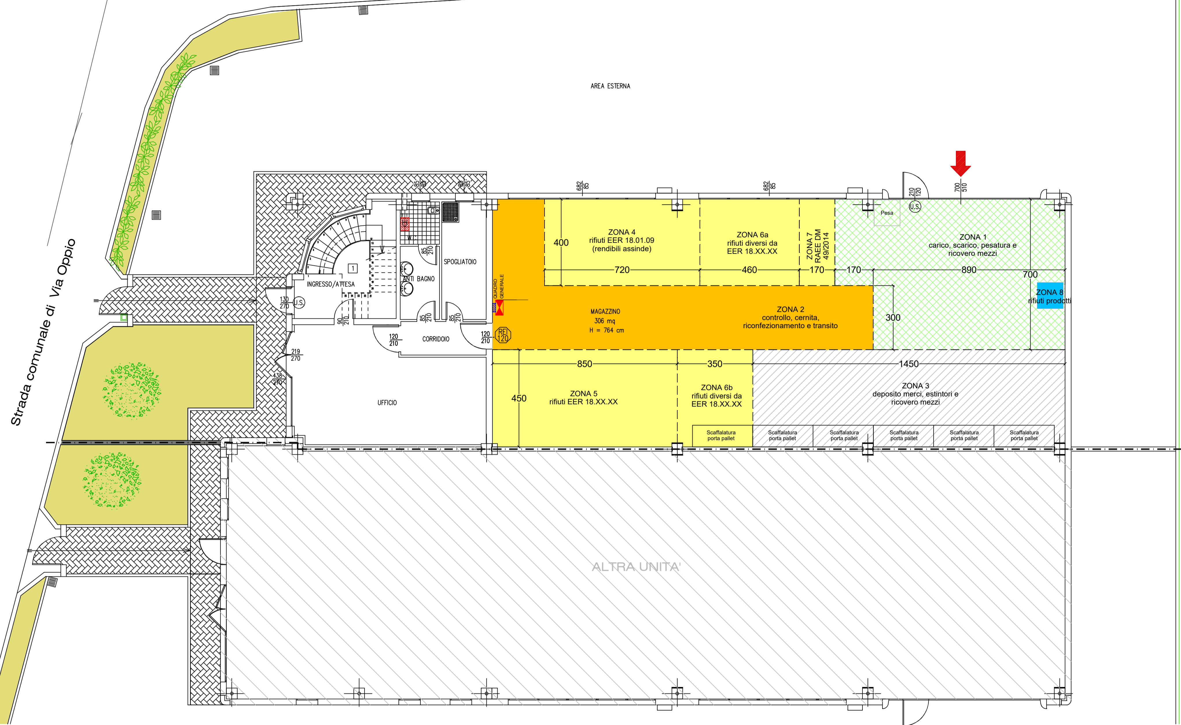
PLANIMETRIA scala 1:100
