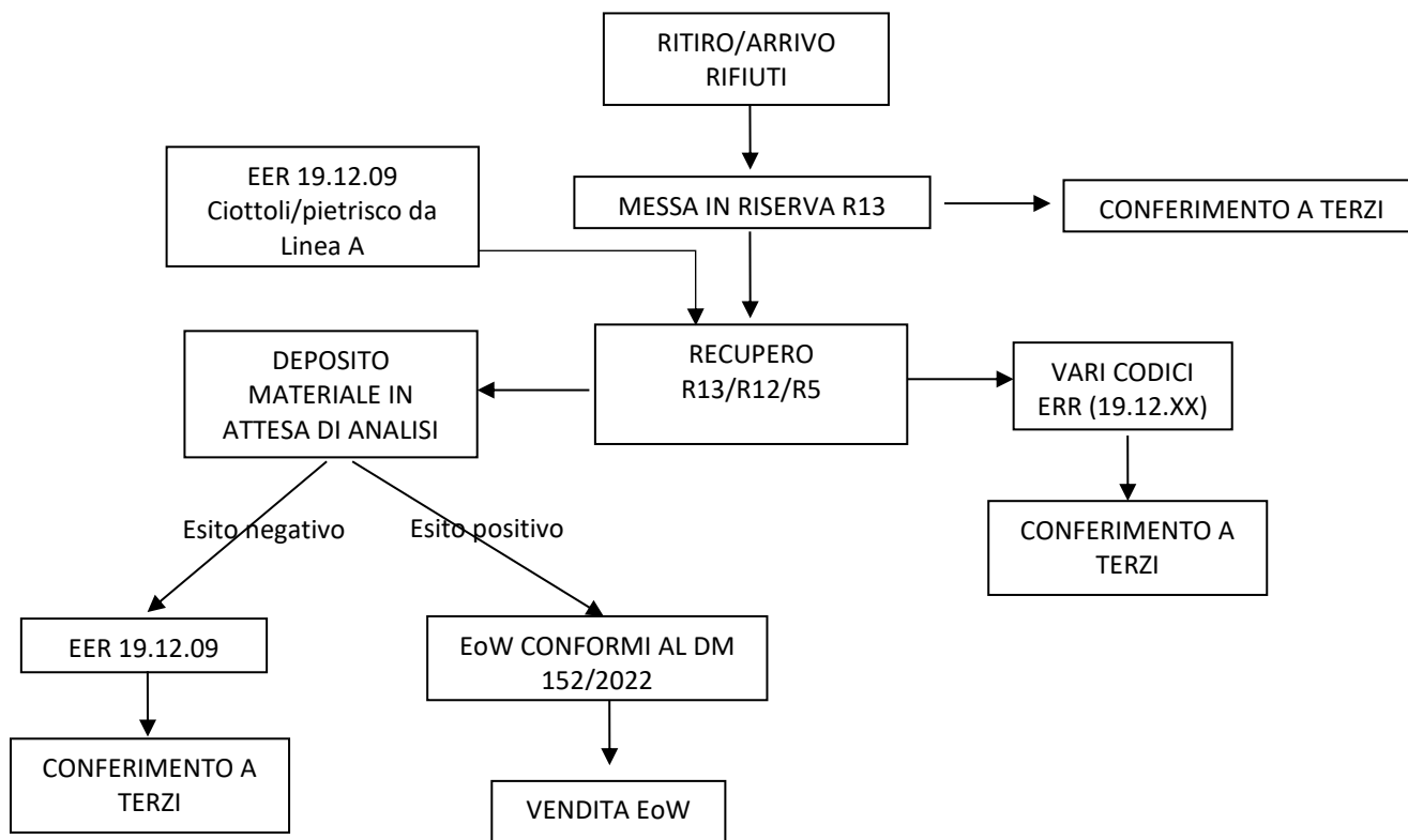
Figura 1. Diagramma di flusso linea B1 EoW Inerti DM 152/2022
